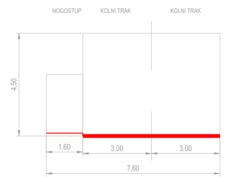
PRESJEK 1-1
