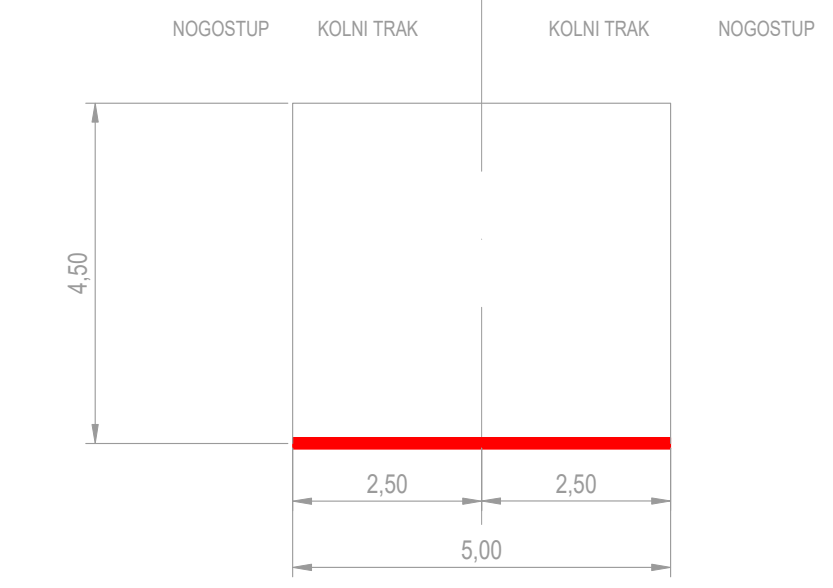
PRESJEK 2-2
